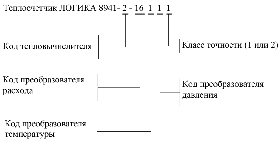
Рисунок 2.1 – Структура обозначения теплосчетчиков
